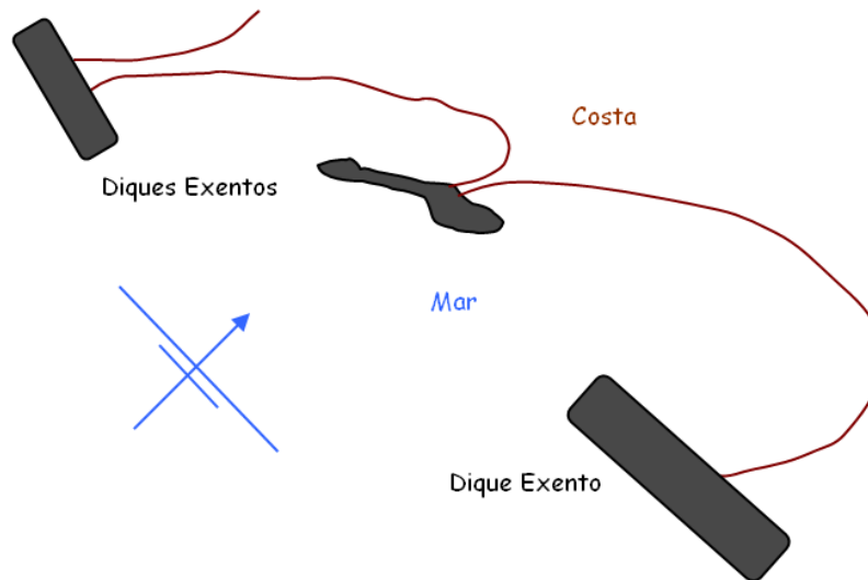
Figura 3.10: Dique Exento
